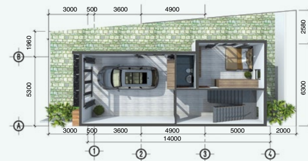
MẶT BẰNG TRỆT
