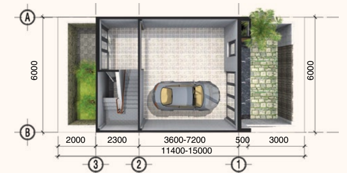
MẶT BẰNG TRỆT
